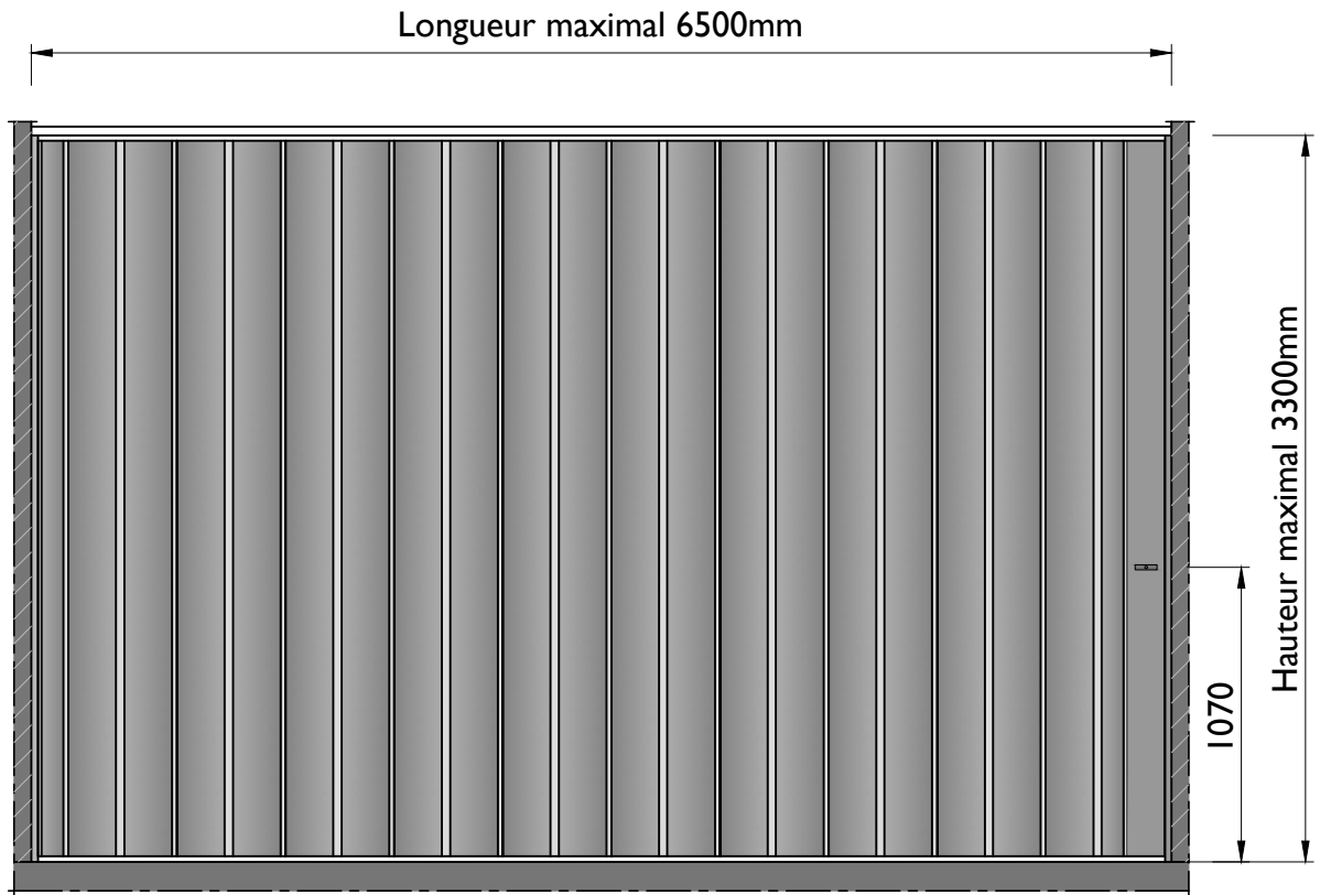
Vue cloison extensible UNO
